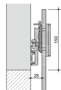
Porte scorrevoli Scorrimento esterno vano Sliding doors - External
