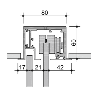
Pareti scorrevoli - Scorrimento interno vano Sliding doors - Internal
