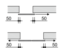
Porte scorrevoli - Scorrimento esterno vano Sliding doors - External
